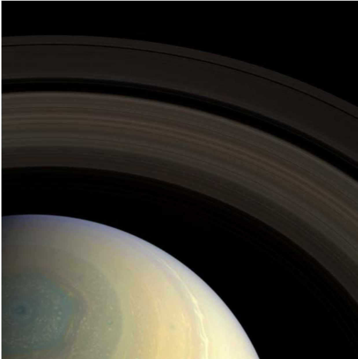
Abbildung 8: Saturns Hexagon
